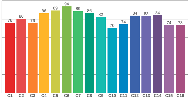
TM30: 81,2
